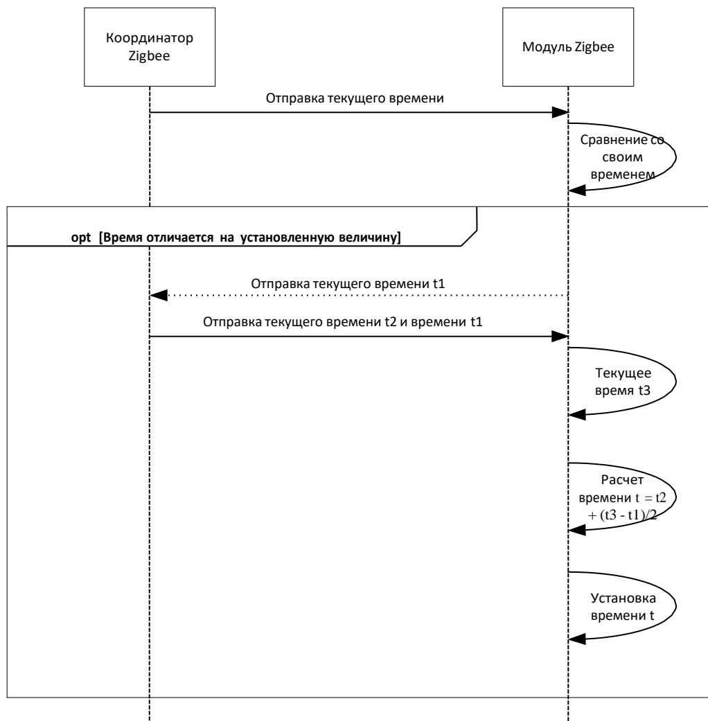
Рисунок 7 – Схема синхронизации времени
